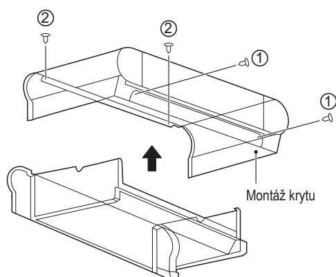
Obrázok 4-4 Demontáž krytu
