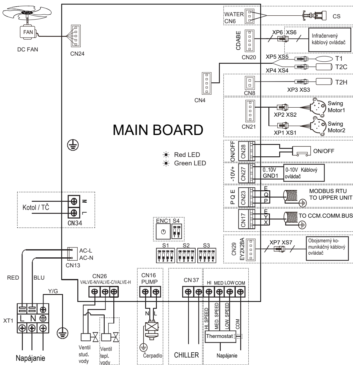
Obrázok 5-20 Schéma zapojenia (jednotka s invertorovým motorom I-VM; I-VN)
