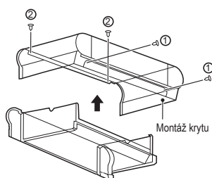
Obrázok 4-6 Demontáž krytu
